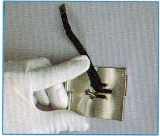
Po wyprostowaniu kabla przełóż śrubę w odpowiednim miejscu
